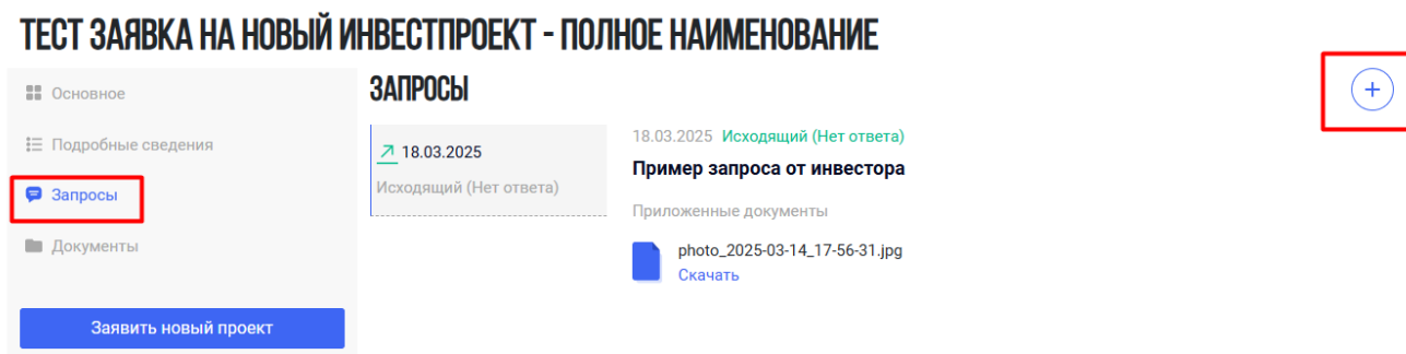
Рисунок 4 – Создание запроса
